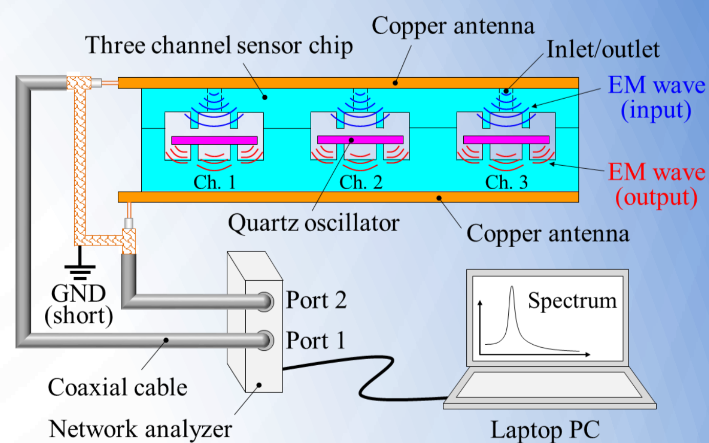
<PDMS-QCM全体図>
